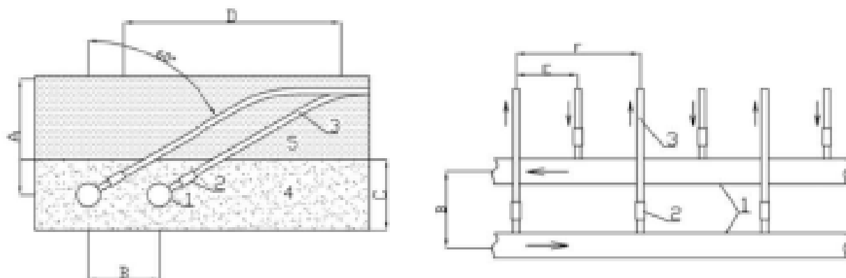
Рис. 2. Одностороннее подключение контуров системы снеготаяния
