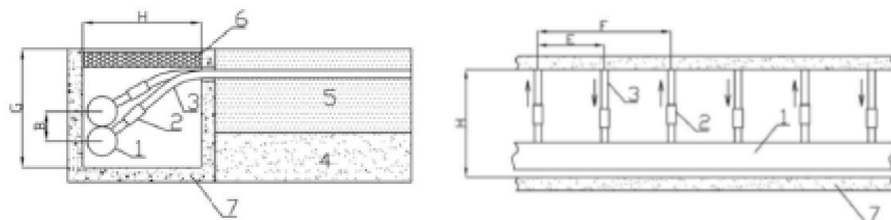
Рис. 3. Подключение к коллектору, расположенному в бетонном кессоне вдоль одной из сторон системы
