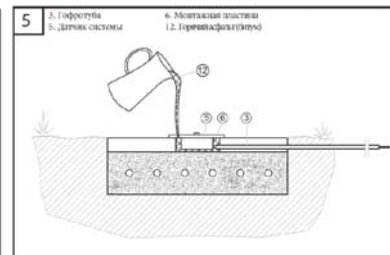
Когда датчик установлен в полости, с помощью монтажной пластины закрепить его горизонтально и вровень с поверхностью. После этого зафиксировать датчик, залив свободное пространство горячим асфальтом или дорожным битумом.
