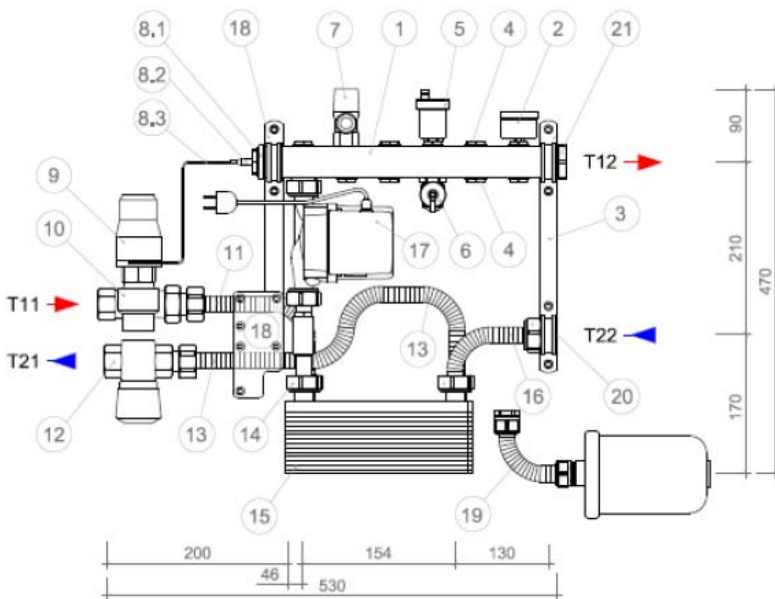
Рис.10. Теплообменный узел ABC серии «Е», компоновка
